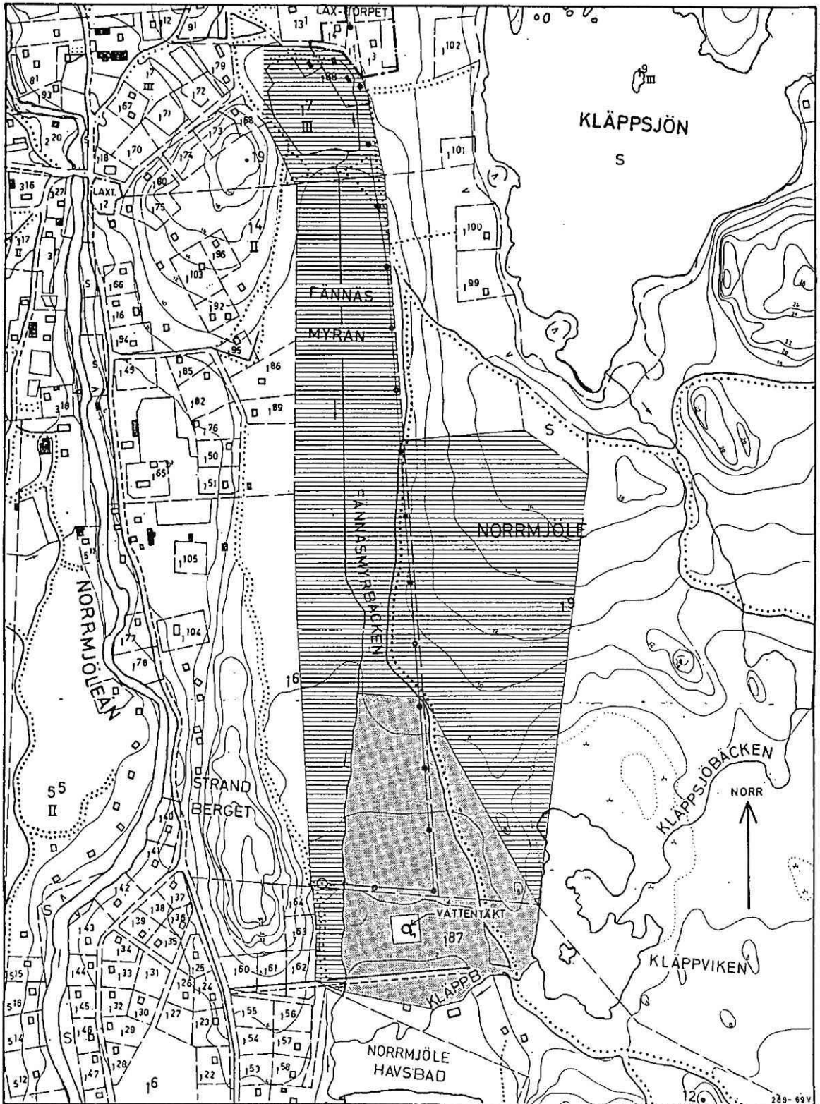
KARTA ÖVER SKYDDSZONER FÖR GRUNDVATTENTILLGÅNG VID NORRMJÖLE HAVSBAD HÖRNEFORS KOMMUN
